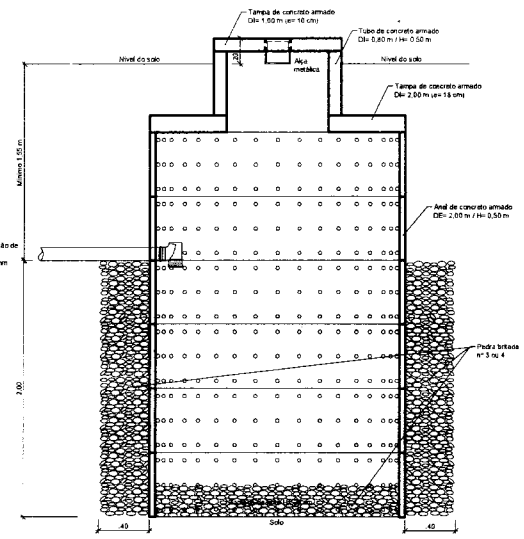
SUMIDOURO - CORTE ESC: 1/20
