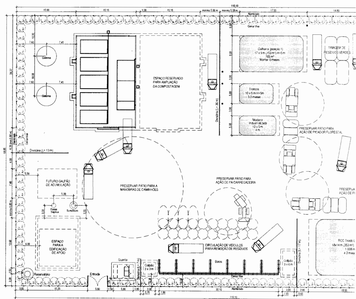
IMPLANTAÇÃO Esc 1:200
