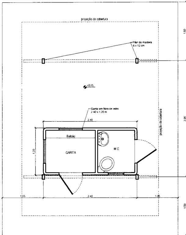
PLANTA ESC. 1/20
