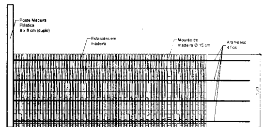
VISTA 1 - CERCA DE ESTACOTE ESC. 1/20
