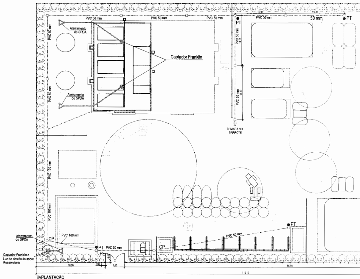
IMPLANTAÇÃO ESC. 1:200
