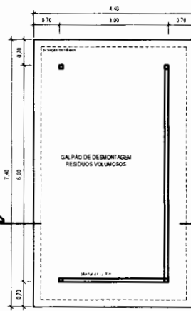
PLANTA
