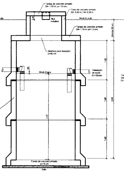
FOSSA SÉPTICA - CORTE ESC: 1/20
