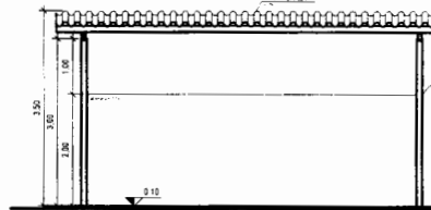
VISTA 1
