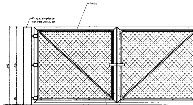
PORTÃO - VISTA FRONTAL ESC. 1/20
