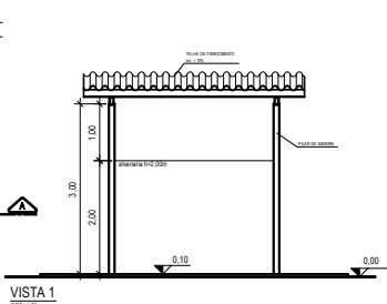
VISTA 1 ESC. 1:50
