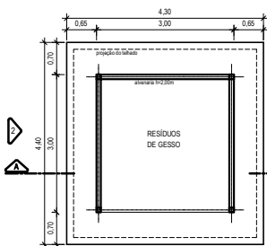
PLANTA ESC. 1:50
