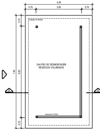
PLANTA ESC. 1:50
