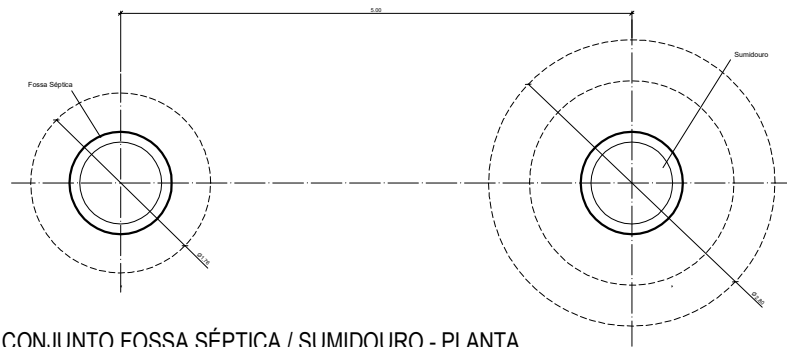
CONJUNTO FOSSA SÉPTICA / SUMIDOURO - PLANTA ESC.1:25
