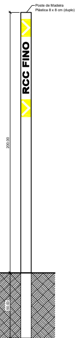
SINALIZAÇÃO VERTICAL esc.: 1:10
