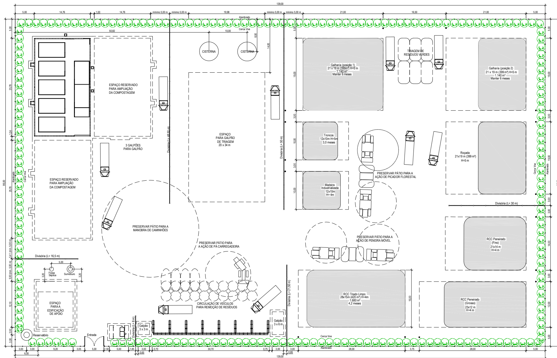
IMPLANTAÇÃO ESC: 1:200
