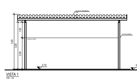
VISTA 1 ESC. 1:50
